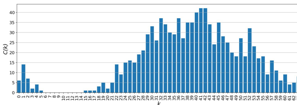
Рисунок 1. Распределение ответов от q -мерного ФНФ ККО
