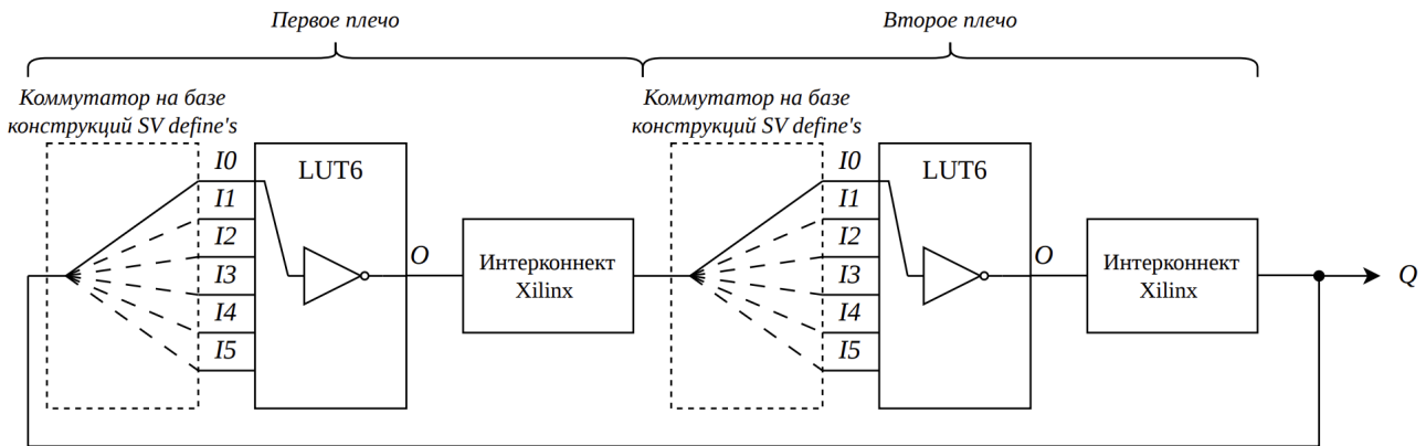
Рисунок 2. Бистабильный элемент на базе примитивов LUT6
