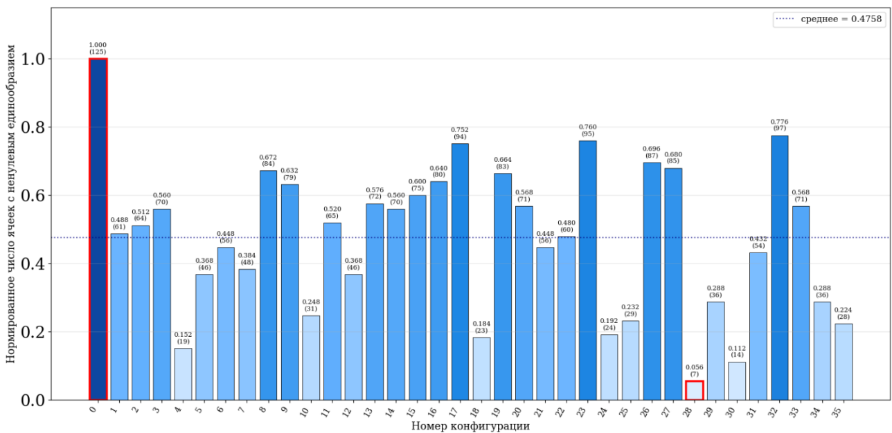
Рисунок 4. Диаграмма распределения нестабильных ячеек по номеру конфигурации
