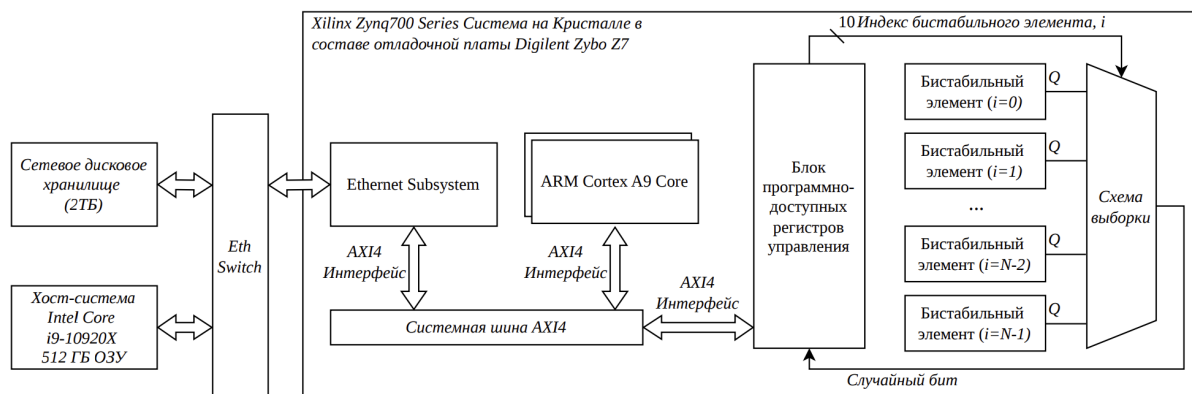
Рисунок 1. Аппаратная платформа для проведения экспериментов
