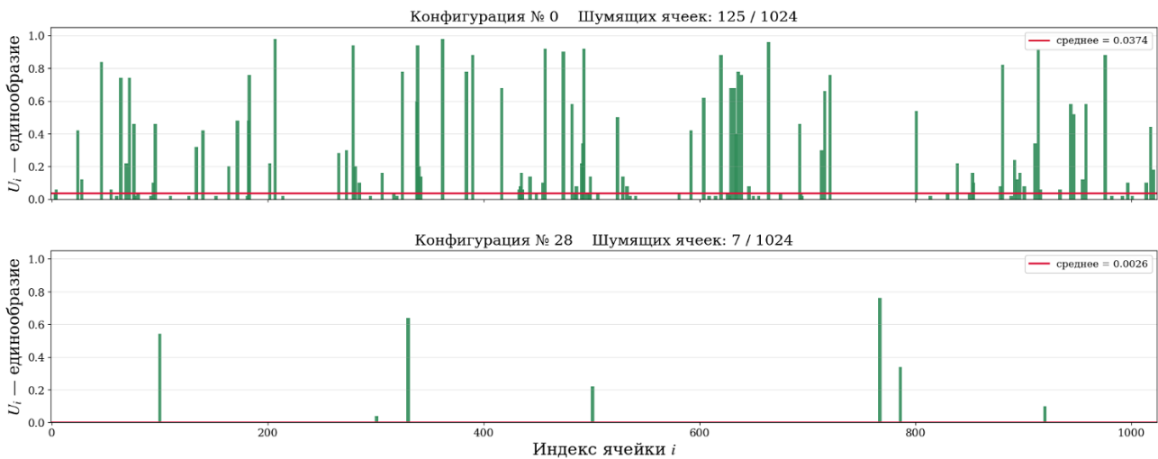
Рисунок 3. Распределение единообразия по ячейкам в разных конфигурациях сетей межсоединений
