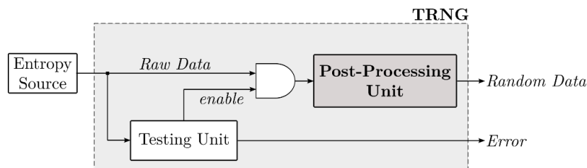
Рис. 1. Обобщенная структура одноканального TRNG
