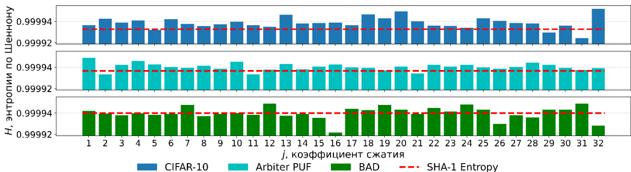
Рис.2 – Энтропия обработанных последовательностей схемой на базе MISA* с различным j
