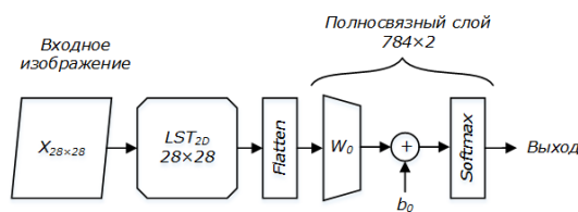
Рисунок 1. Архитектура LST-1
