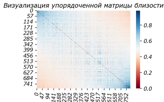
Рисунок 2. Упорядоченная матрица сходства признаков LST-слоя
