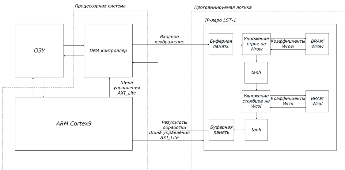
Рисунок 4. Структурная схема аппаратно-программной реализации (вариант В)
