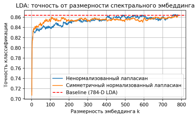
Рисунок 3. Зависимость точности классификации от размерности спектрального эмбединга для комбинаторного и нормализованного лапласианов
