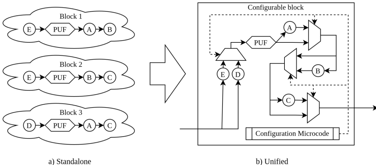
Рисунок 1. Пример перехода от архитектуры с разделяемыми функциями к архитектуре с реконfigurацией аппаратуры и переиспользованием аппаратных блоков
